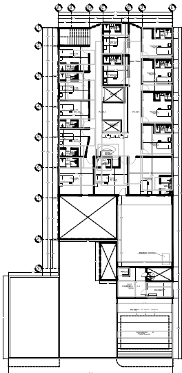
PLANTA SEGUNDO NIVEL CLÍNICA DEL CONCHI
